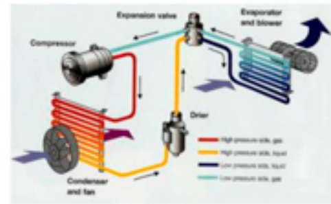
วงจรเครื่องปรับอากาศรถยนต์
