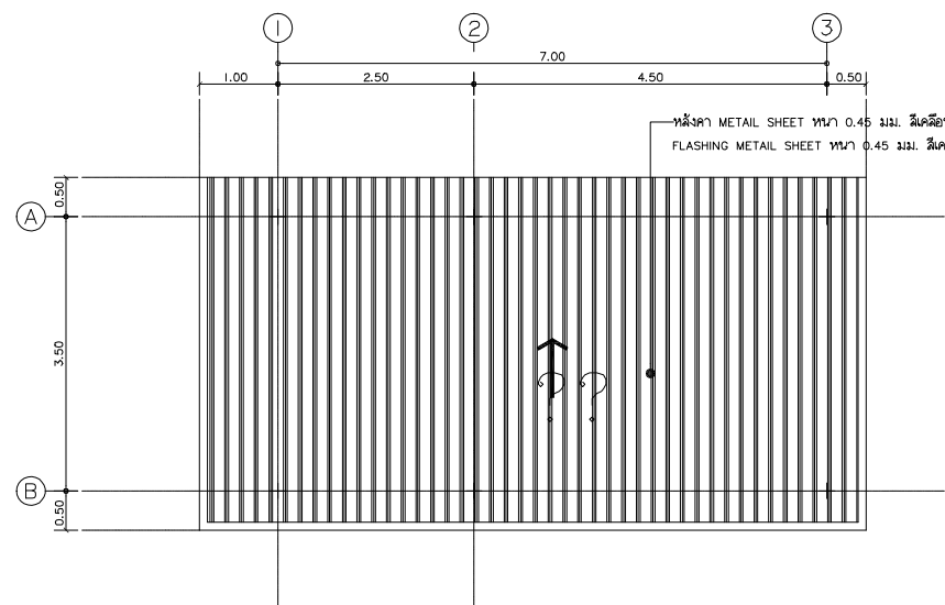
แปลนหลังคา SCALE 1:50
