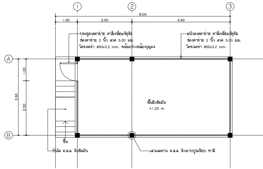
แปลนพื้น (+ 1.20 m.) SCALE 1:50
