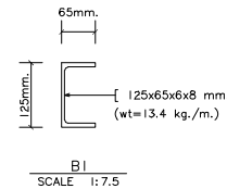
รายละเอียดคาน BI เหนือ Grid line E, F, G SCALE 1:7.5
