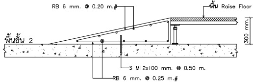
รายละเอียด Ramp ทางขึ้นพื้น Raise Floor SCALE 1:20
