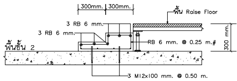
รายละเอียดบันได ทางขึ้นพื้น Raise Floor SCALE 1:20
