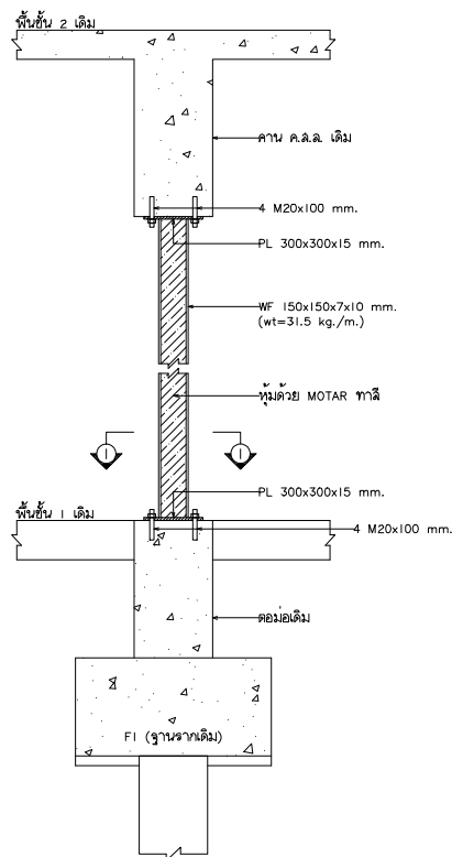
รายละเอียดการเสริมเสาเหล็กใต้พื้นชั้น 2 SCALE 1:20
