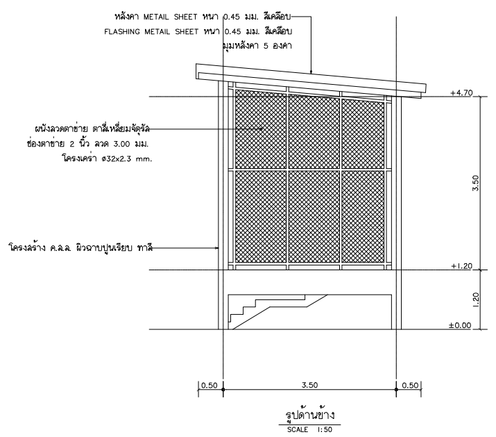
รูปด้านข้าง SCALE 1:50
