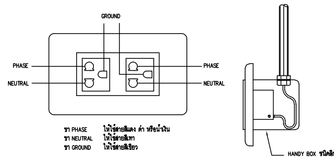
ข้อกำหนดการต่อลงจรของตัวรับไฟฟ้า
