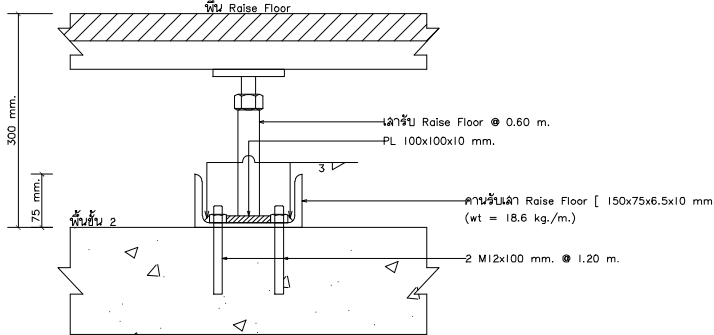
รายละเอียดการเชื่อมยึดคานเหล็ก รับเสา Raise Floor (FS1000) SCALE 1:5
