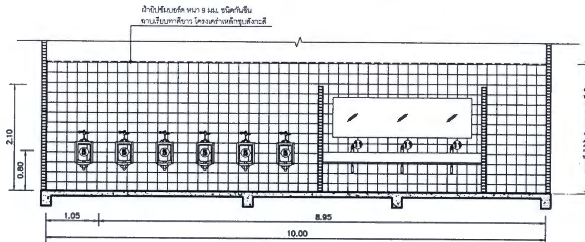
รูปตัดห้องน้ำชาย ชั้น 1
