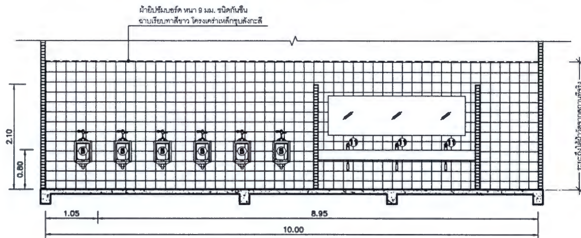
รูปตัดห้องน้ำชาย ชั้น 2
