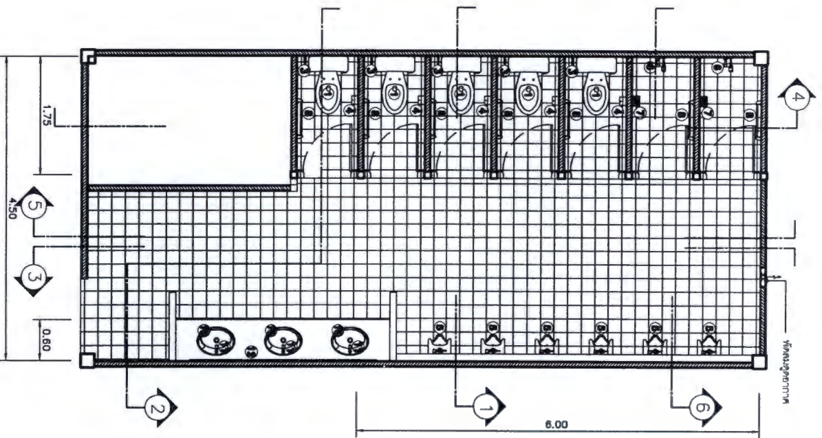
ขยบายรูปห้องน้ำชาย ชั้น 1 มาตราส่วน 1:50
