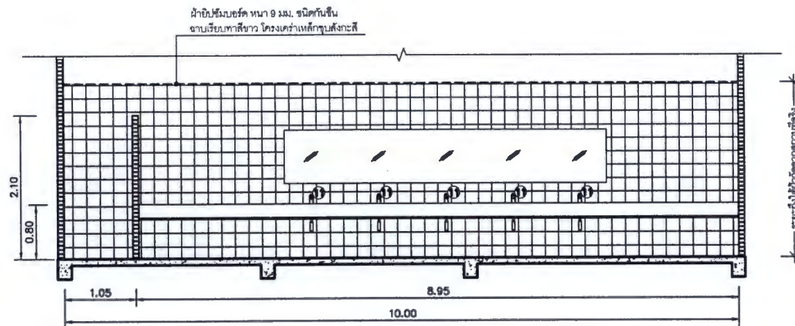
รูปตัดห้องน้ำหญิง ชั้น 2 มาตราส่วน 1:50 ③
