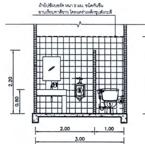
รูปตัดห้องน้ำชาย ด้านหน้า ชั้น 1
