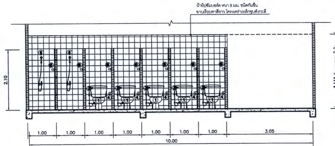
รูปตัดห้องน้ำหญิง ชั้น 2 มาตราส่วน 1:50 ④
