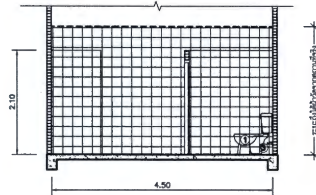
รูปตัดห้องน้ำหญิง ชั้น 1 มาตราส่วน 1:50
