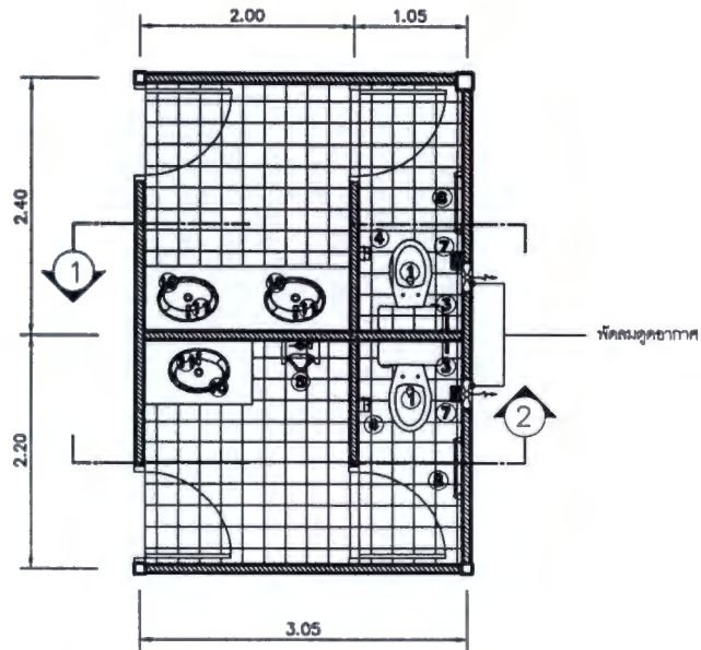
ขยายปรับปรุงห้องน้ำชาย-หญิง ด้านหน้า ชั้น 1 มาตราส่วน 1:50
