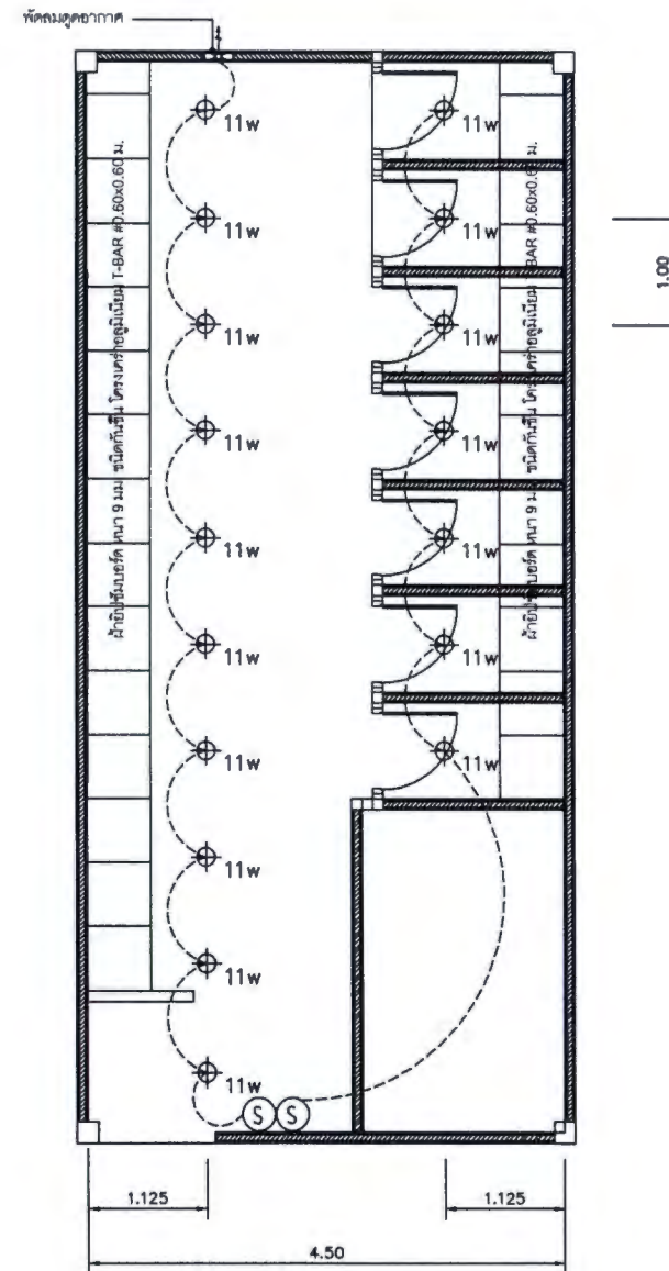
แปลนไฟฟ้าแสงสว่างห้องน้ำหญิง ชั้น 1 มาตราส่วน 1:50
