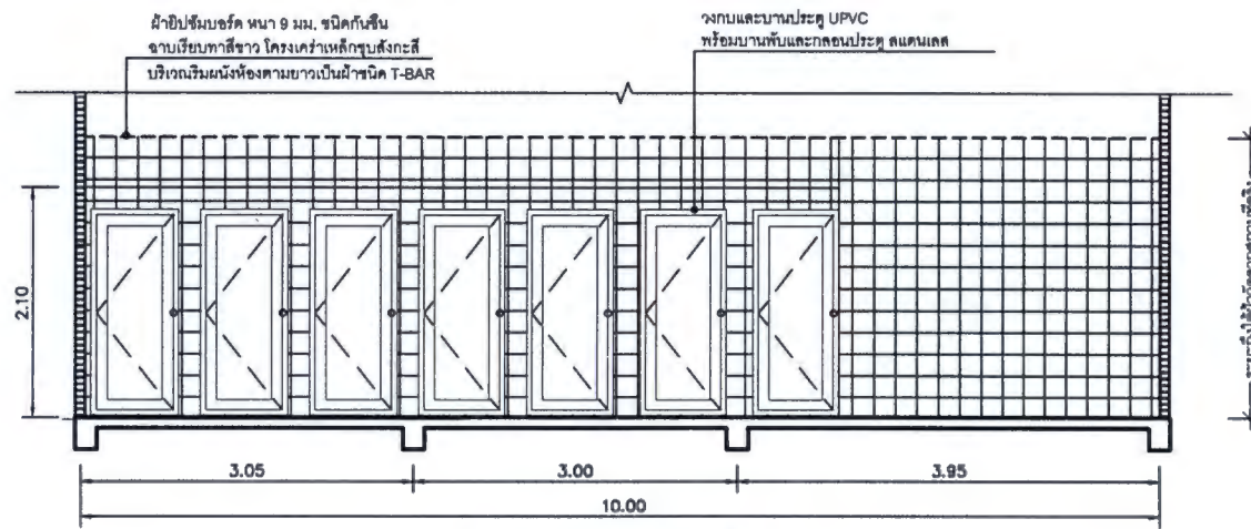
รูปตัดห้องน้ำหญิง ชั้น 1 มาตรฐาน 1:50 5
