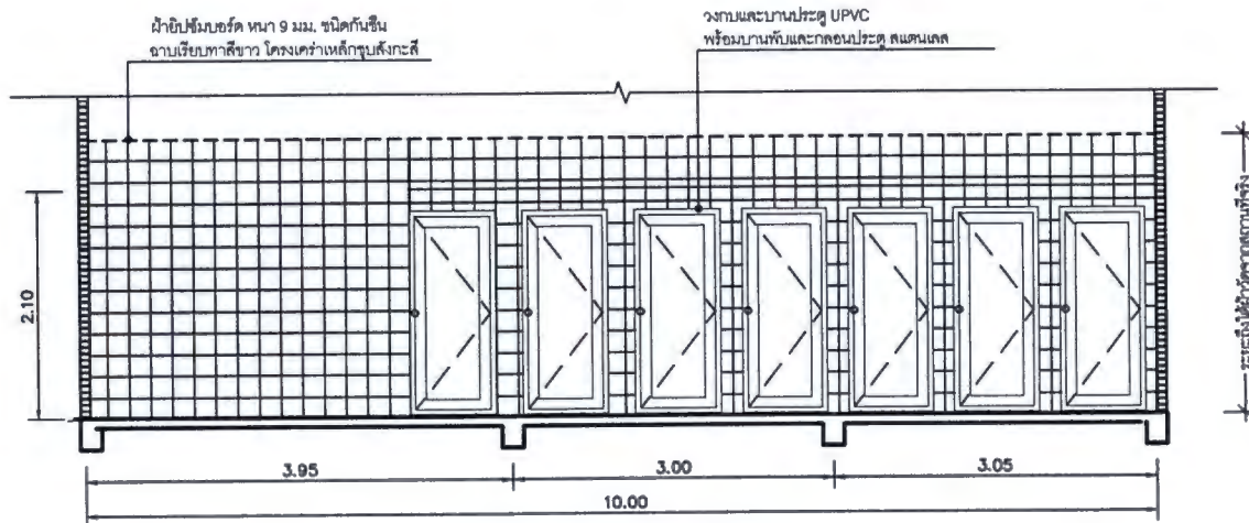
รูปตัดห้องน้ำชาย ชั้น 2 มาตราส่วน 1:50
