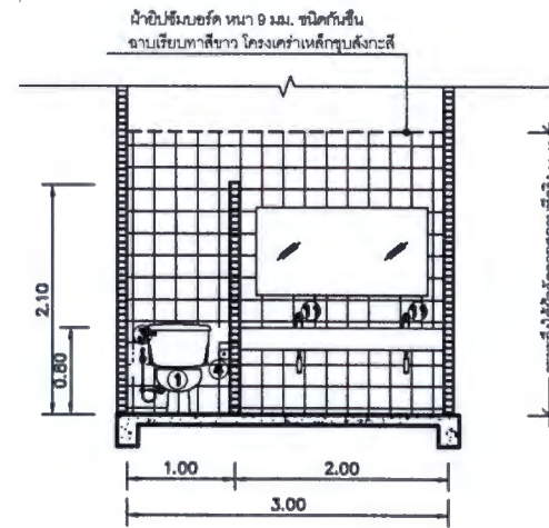
รูปตัดห้องน้ำหญิง ด้านหน้า ชั้น 1
