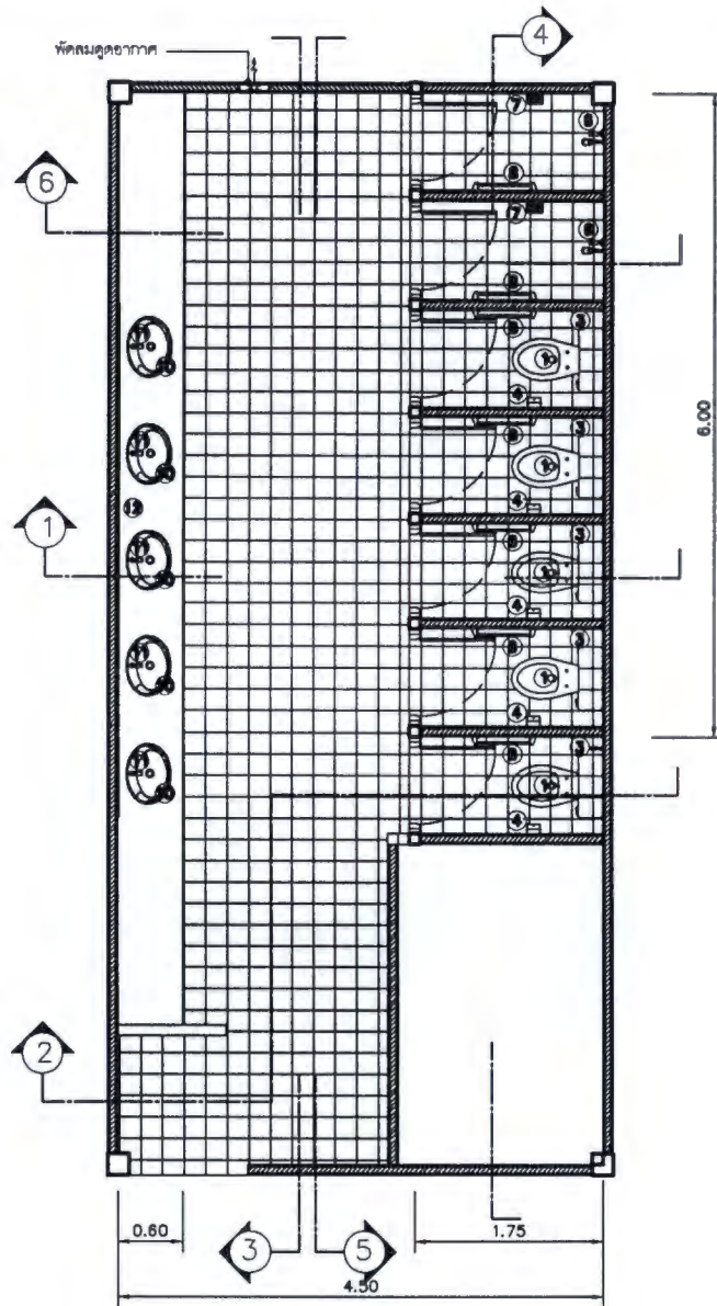
ขยายปรับปรุงห้องน้ำหญิง ชั้น 1 มาตราส่วน 1:50
