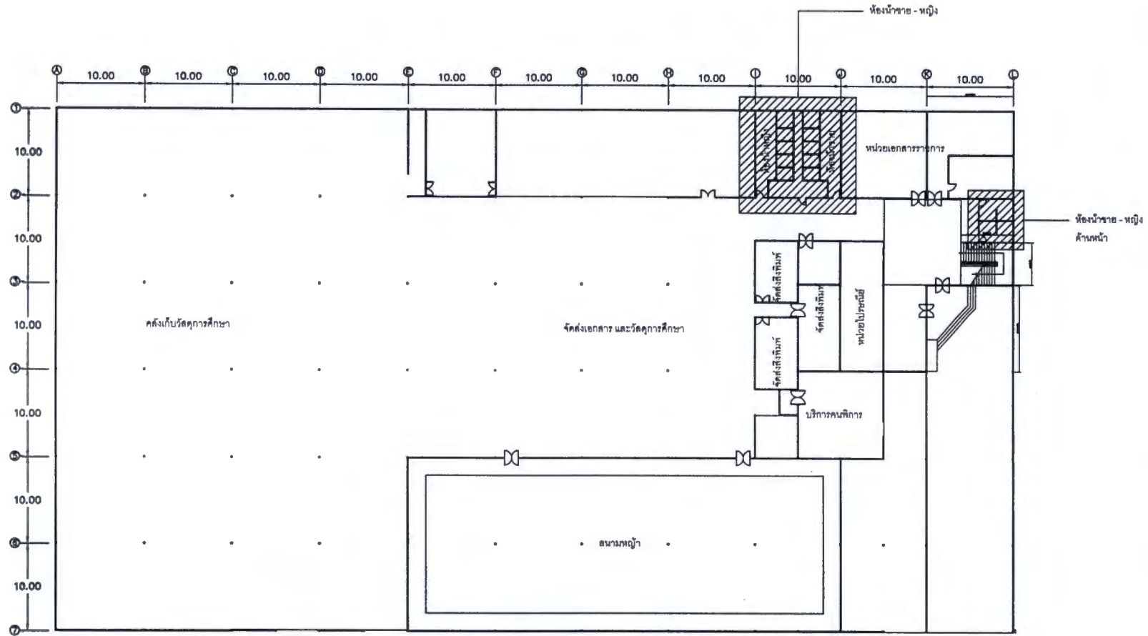
แบบแสดงตำแหน่งการปรับปรุงห้องน้ำ ชั้น 1 มาตราส่วน 1:400
