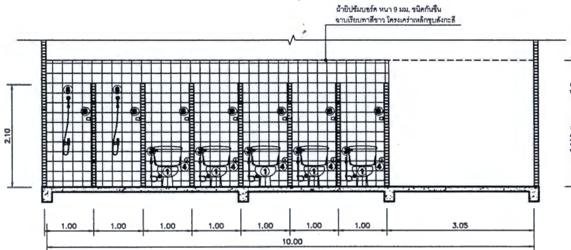
รูปตัดห้องน้ำหญิง ชั้น 1 มาตราส่วน 1:50
