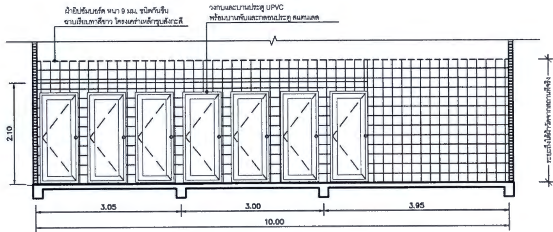
รูปตัดห้องน้ำหญิง ชั้น 2 มาตราส่วน 1:50
