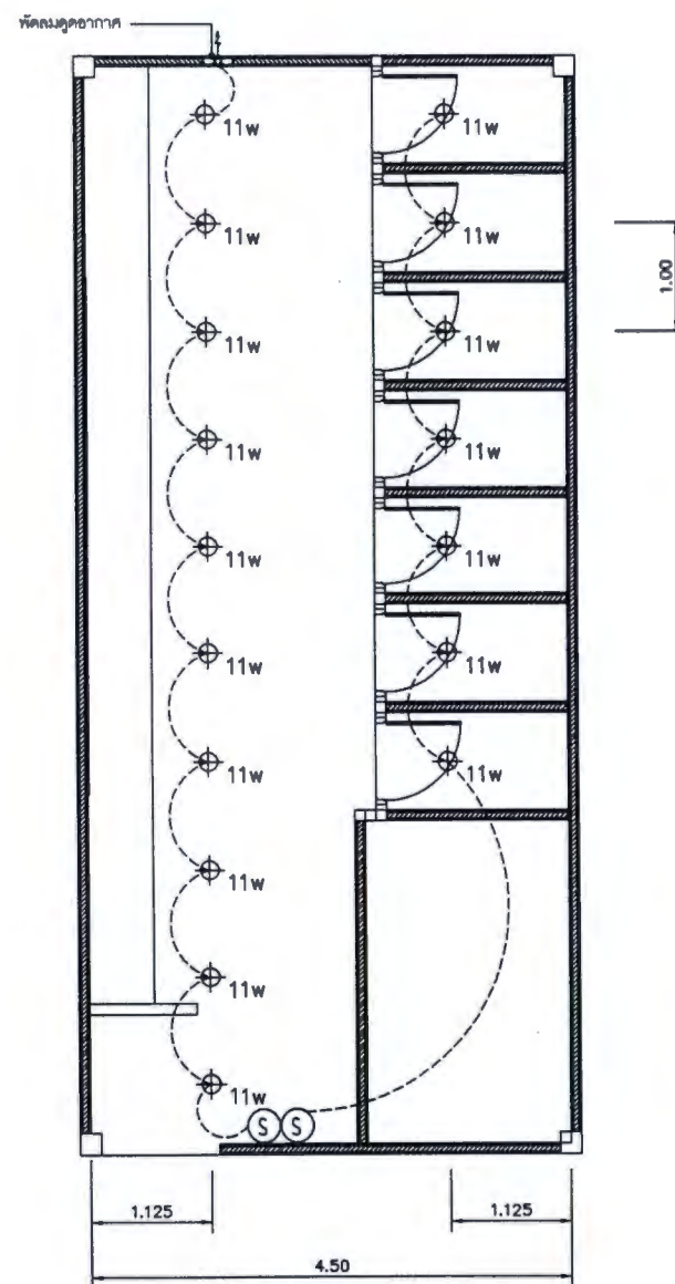
แปลนไฟฟ้าแสงสว่างห้องน้ำหญิง ชั้น 2 มาตราส่วน 1:50
