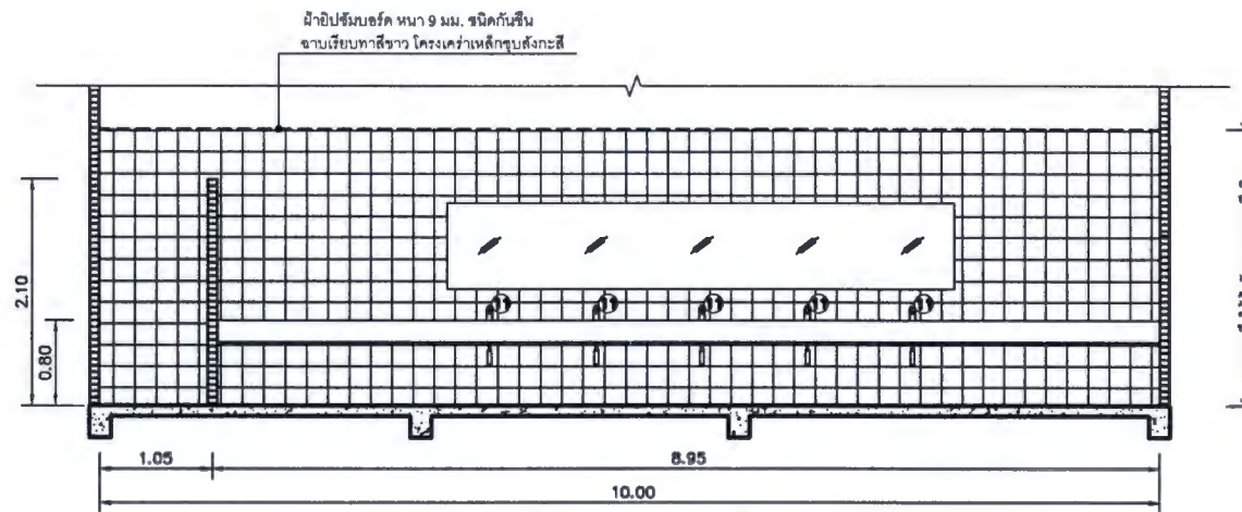
รูปตัดห้องน้ำหญิง ชั้น 1 มาตราส่วน 1:50
