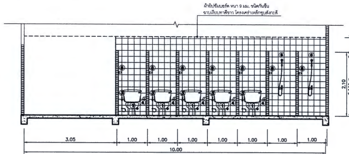
รูปตัดห้องน้ำชาย ชั้น 1
