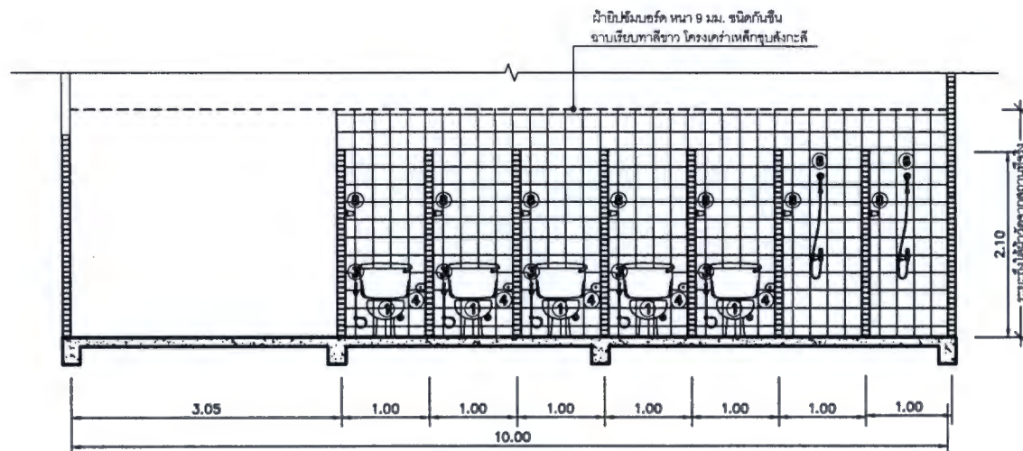
รูปตัดห้องน้ำชาย ชั้น 2
