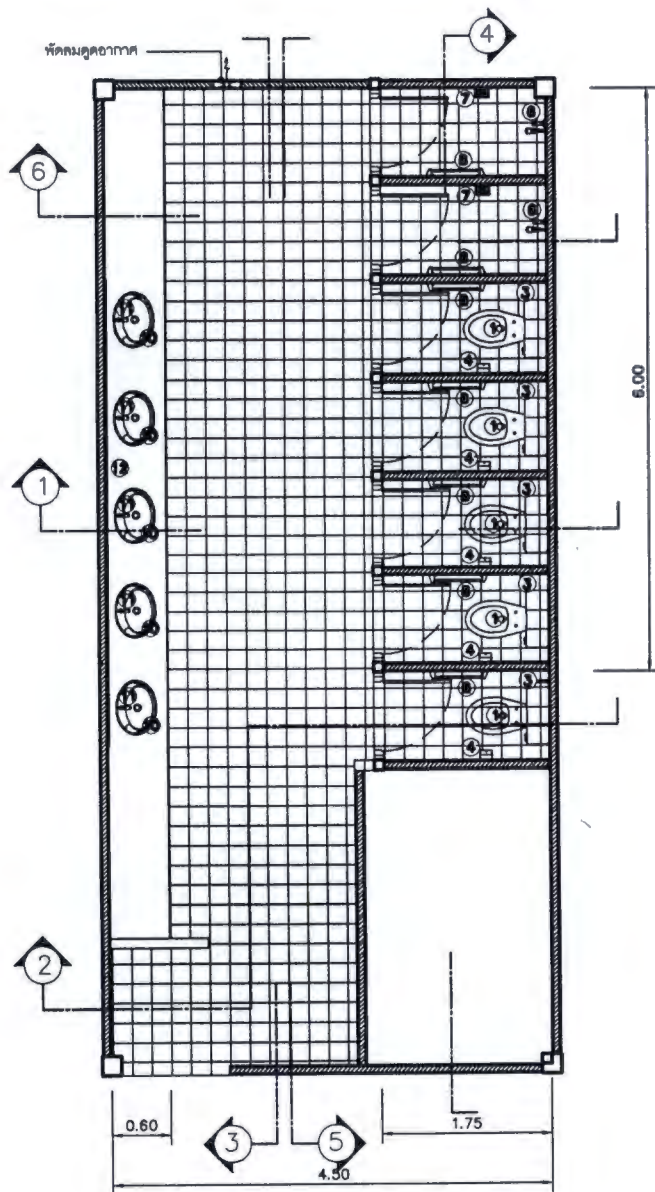
ขยายปรับปรุงห้องน้ำหญิง ชั้น 2 มาตราส่วน 1:50
