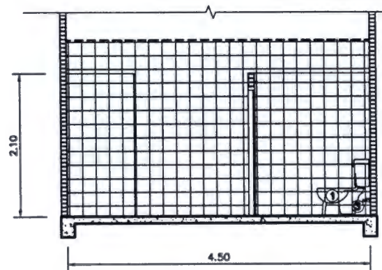
รูปตัดห้องน้ำหญิง ชั้น 2 มาตราส่วน 1:50
