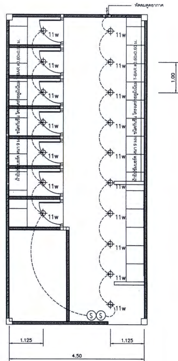
แปลนไฟฟ้าแสงสว่างห้องน้ำชาย ชั้น 1
